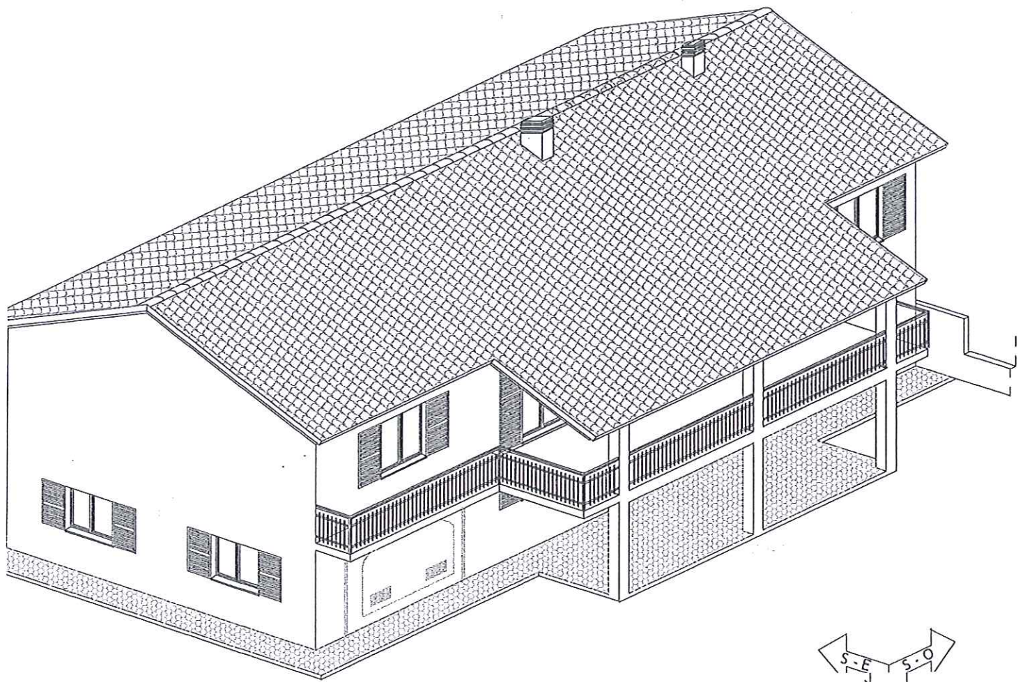
VISTA ASSONOMETRIC.
